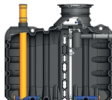
Et minirensningsanlæg
